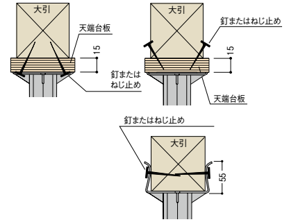
〔フクビ〕 プラ束宝生 台板タイプ (木造軸組工法の場合)プラ束間隔・大引き間隔 1000mm以内
