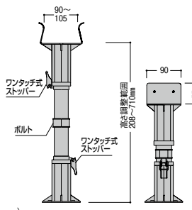
〔フクビ〕 プラ束宝生 受座タイプ (木造軸組工法の場合)プラ束間隔・大引き間隔 1000mm以内
