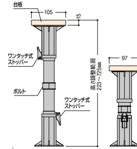
〔フクビ〕 プラ束宝生 台板タイプ (木造軸組工法の場合)プラ束間隔・大引き間隔 1000mm以内
